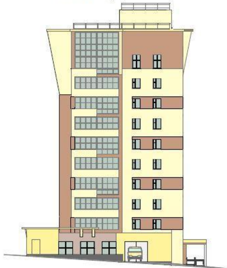
ВОСТОЧНЫЙ ФАСАД
